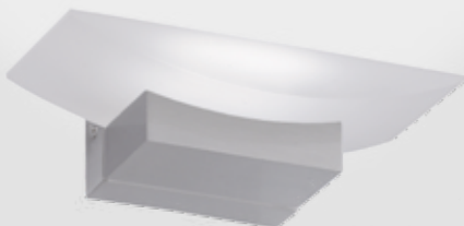
2628421. nickelfarben matt, Acrylglas satiniert, über Taster stufenlos dimmbar und tunable white(cct) in 3 Stufen einstellbar, 6,5 W LED, 2700/3350/4000 K, 610 lm, B 200, H 70, A 110 € 116,50
